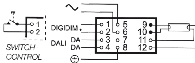
Schéma zapojení EL-si Wiring diagram EL-si
